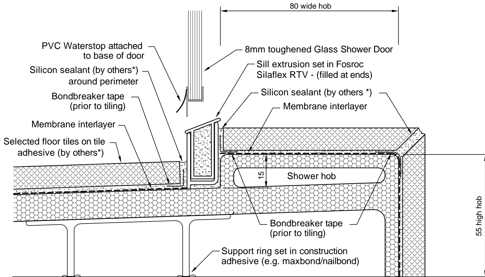
DETAIL 2 HOB TRAY DOOR SILL 01
